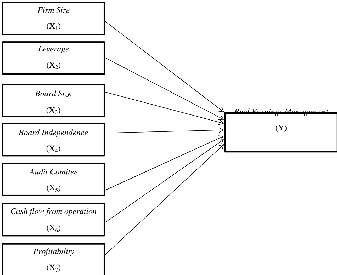
Gambar 1. Kerangka Pemikiran
