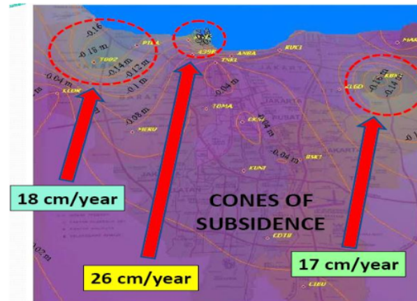
Gambar 4, Penurunan muka tanah di DKI Jakarta Sumber Hasanudin, 2008. Dalam Ali. F. 2009.
