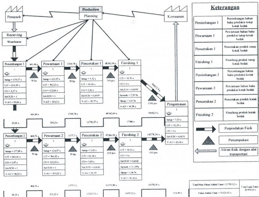
Gambar 3 Current Value Stream Map Proses Produksi untuk Produk Set Kotak bedak.
