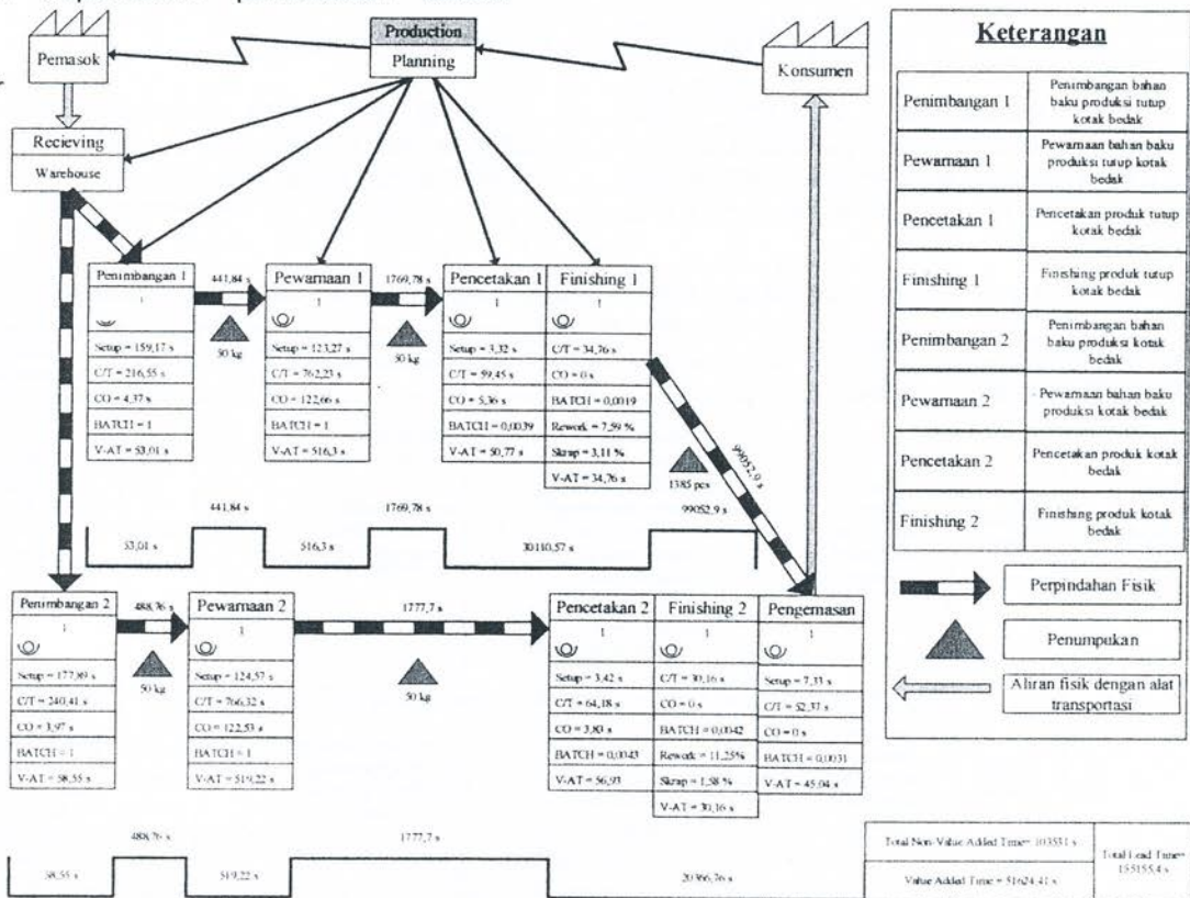
Gambar 9. Future Value Stream Map Proses Produksi untuk Produk Set Kotak Bedak
