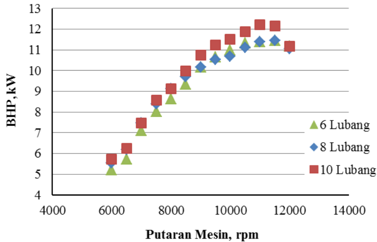
Gambar 2. BHP terhadap putaran mesin
