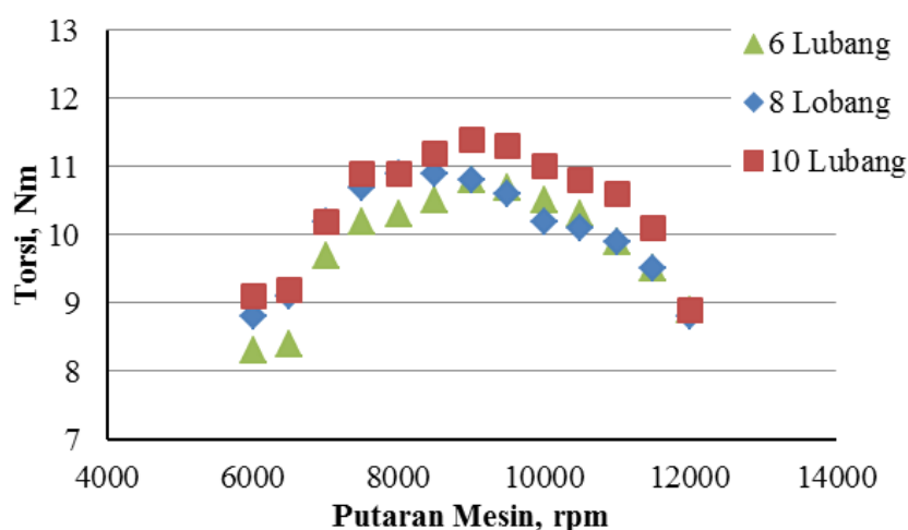
Gambar 1. Torsi terhadap putaran mesin
