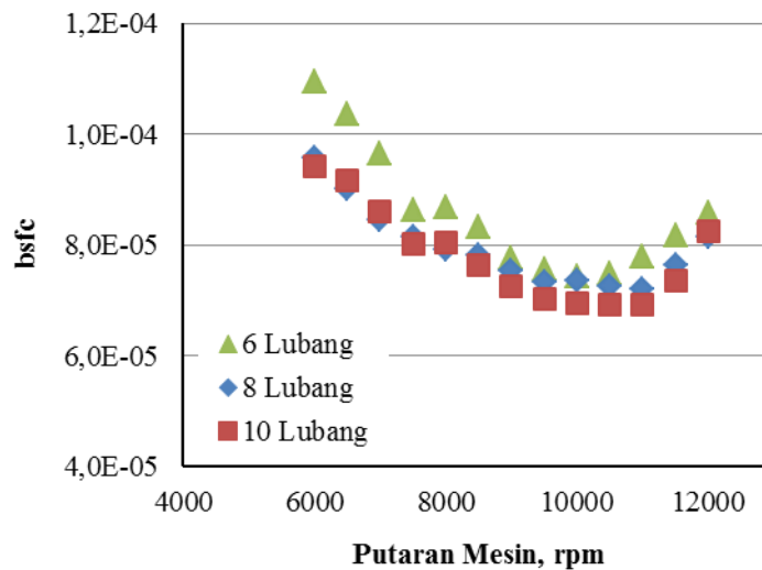
Gambar 4. BSFC terhadap putaran mesin
