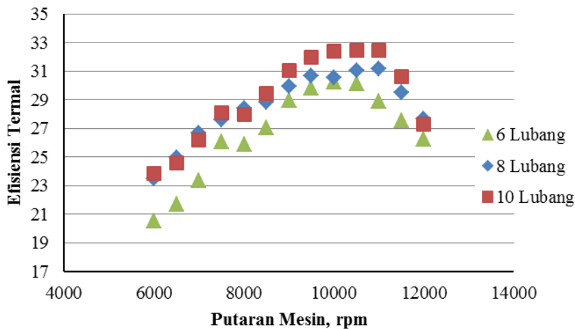
Gambar 3. Efisiensi termal terhadap putaran mesin
