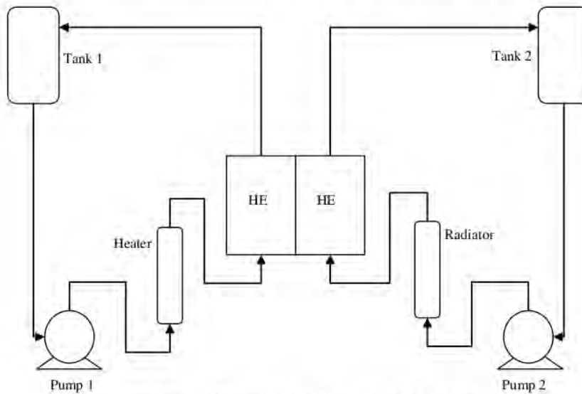
Gambar 1. Sistem instalasi Alat Penukar Kalor
