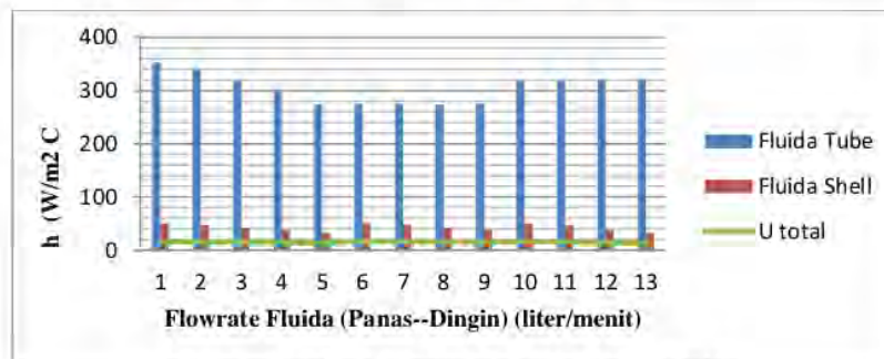
Gambar 2. Koefisien Perpindahan Panas Fluida
