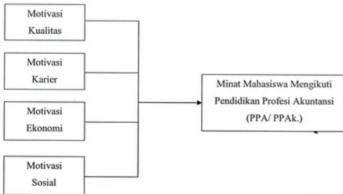
Gambar 1. Kerangka Penelitian
