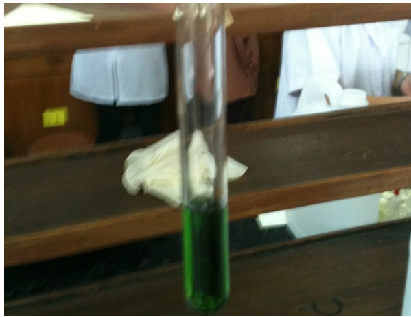
Gambar 3.1 Penambahan H_2SO_4 2N
