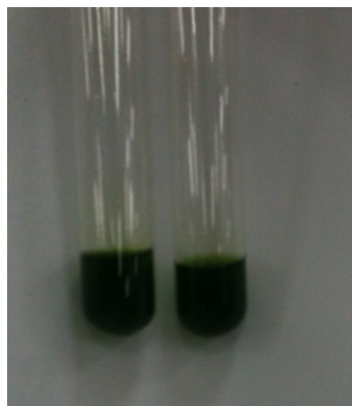
Gambar 3.3 Tabung Uji dan Tabung Kontrol
