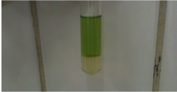
Gambar 3.4 Setelah Ditambahkan NaOH 10%
