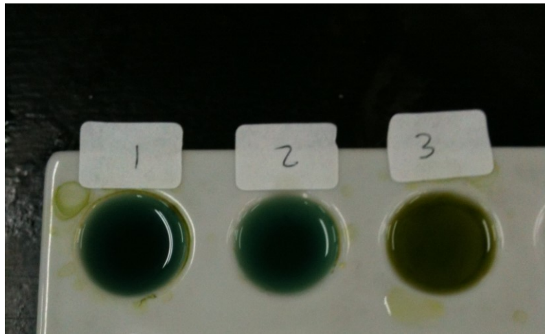
Gambar 4.5 Hasil Uji Steroid dan Triterpenoid Sampel Segar
