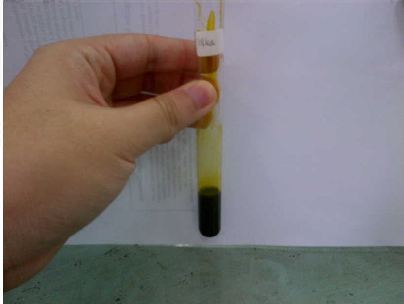
Gambar 3.7 Setelah Ditambahkan Kloroform dan Amoniak
