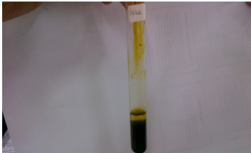
Gambar 3.8 Setelah Ditambahkan H_2SO_4
