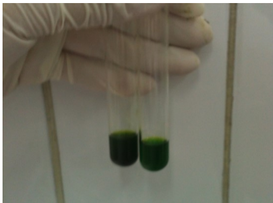
Gambar 4.2 Hasil Uji Fenolik Sampel Segar
