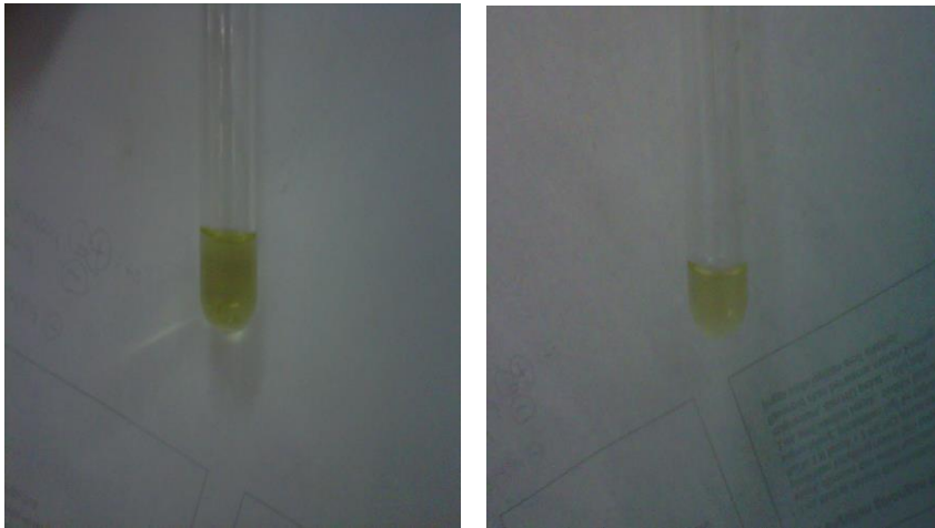
Gambar Hasil Pengujian Golongan Alkaloid pada Sampel Kering (Kiri Dengan Pereaksi Mayer Tidak Terbentuk Endapan Putih dan Kanan Dengan Pereaksi Dragendorff Tidak Terbentuk Endapan Jingga)
