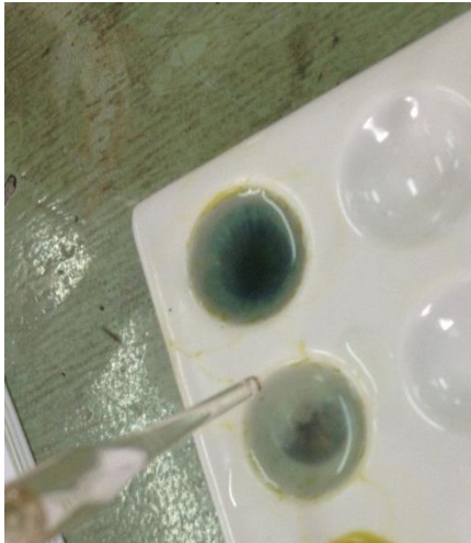
Uji Steroid
