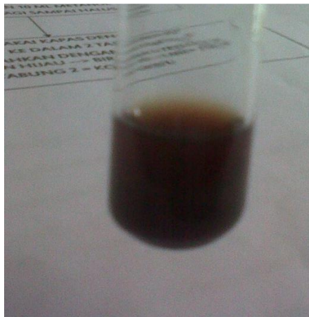
Uji Fenolik
