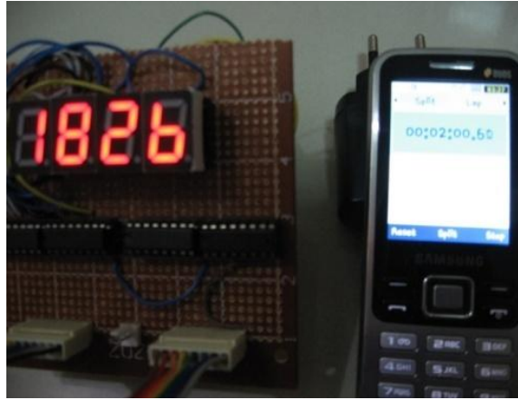
■ Gambar 10. Hasil Pengujian RTC DS1307 Setelah Dua Menit
