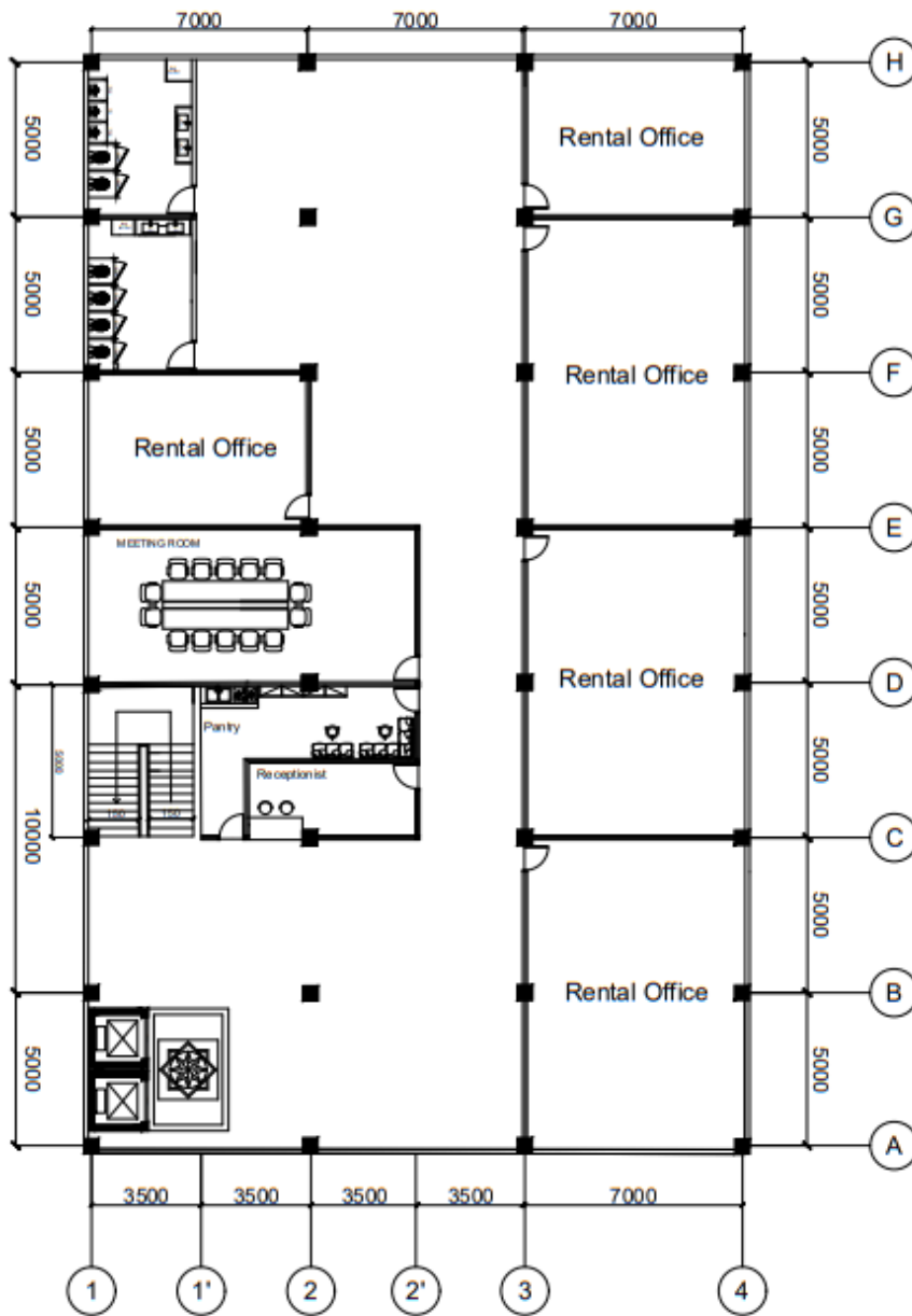
Gambar 1. Denah bangunan
