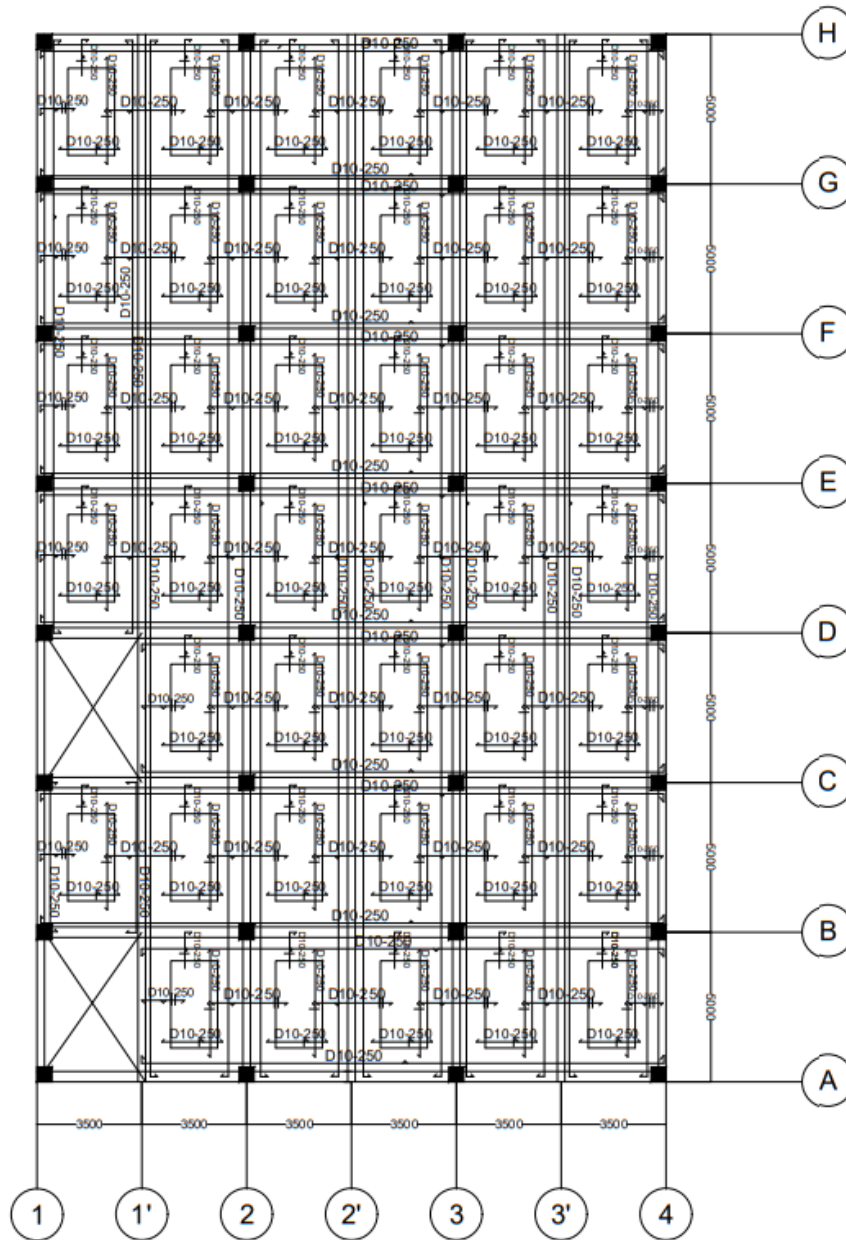
Gambar 2. Denah penulangan pelat lantai
