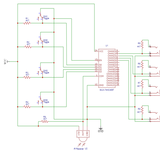
Gambar 5. Skematik Diagram
