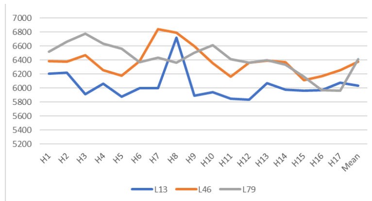
Gambar 2. Data rata-rata tingkat pencahayaan (lux) ke tiga set lampu dengan waktu jeda 1 detik terhadap hari pengukuran
