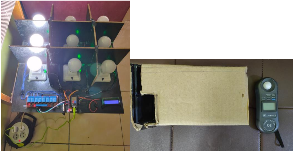
Gambar 1. Alat Ukur umur lampu dengan teknologi switching cycle
