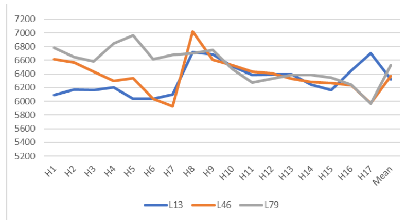
Gambar 3. Data rata-rata tingkat pencahayaan (lux) ke tiga set lampu dengan waktu jeda 4 detik terhadap hari pengukuran
