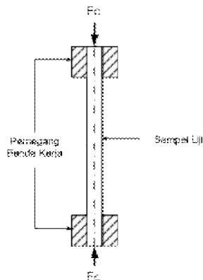
Gambar 1 Skema pengujian tekan
