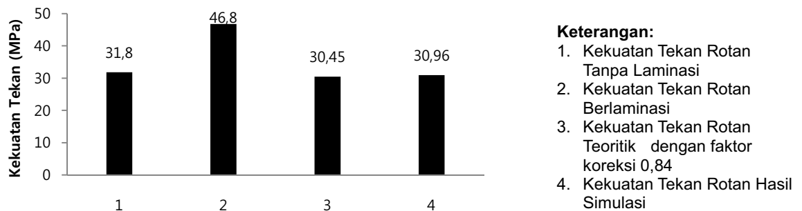
Gambar 3 Grafik perbandingan kekuatan tekan
