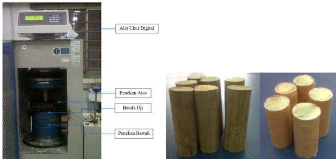
Gambar 4 Alat uji tekan dan posisi benda uji
