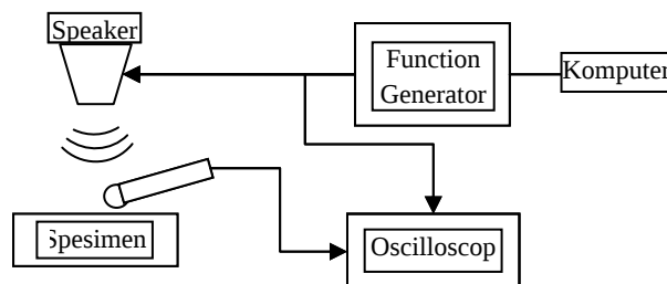
Gambar 1. Eksperimental set - up
