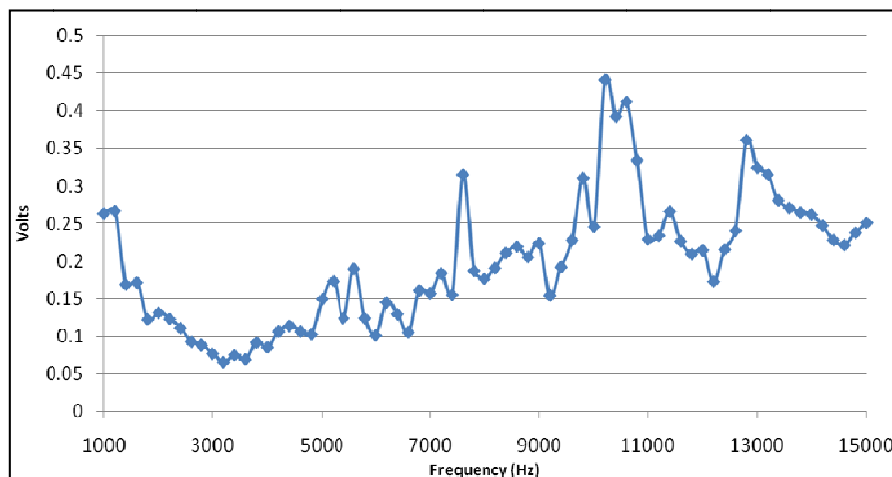
Gambar 4. Grafik distribusi Tingkat Tekanan Bunyi pada 80 dB
