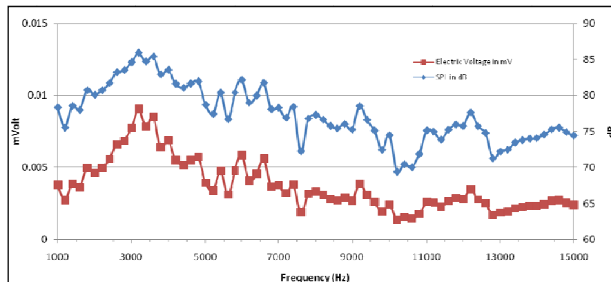
Gambar 3. Hasil keluaran dari Sound Level Metre (SLM)
