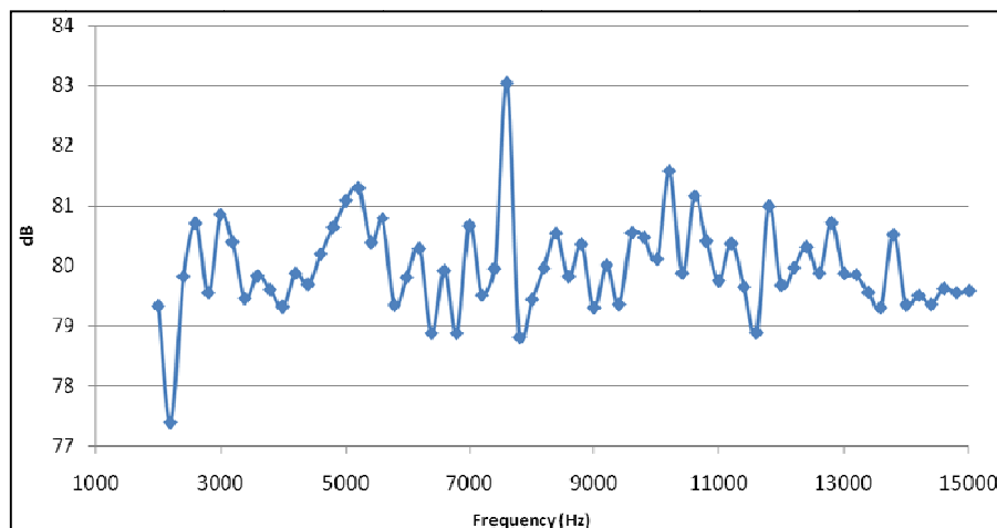
Gambar 5. Grafik Tekanan Bunyi dengan pengaturan tegangan
