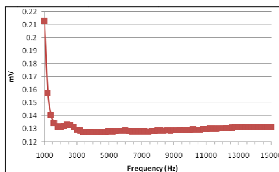
Gambar 2. Tegangan masukan terukur speaker
