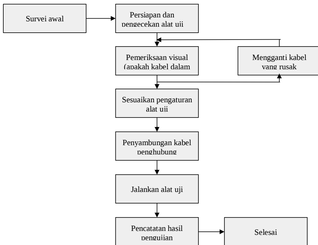
Gambar 6. Diagram Alir Tes Megger
